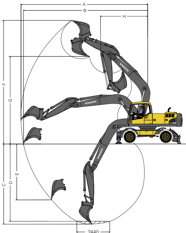
Pluma monobloque de 5,6 m y brazo de 2,45 m, 2,6 m, 2,90 m
