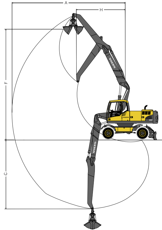
Pluma articulada de 5,5 m y brazo de bivalva de 3,2 m
