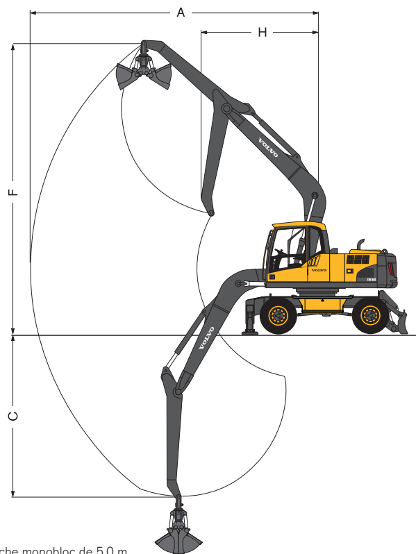
Flèche monobloc de 5,0 m et balancier de 2,95 m pour pince
