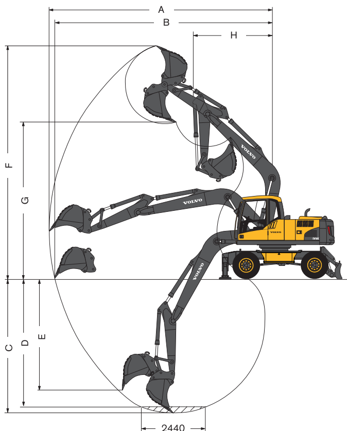
Flèche monobloc de 5,0 m et balancier de 2,0 m, 2,45 m, 2,6 m, 3,1 m
