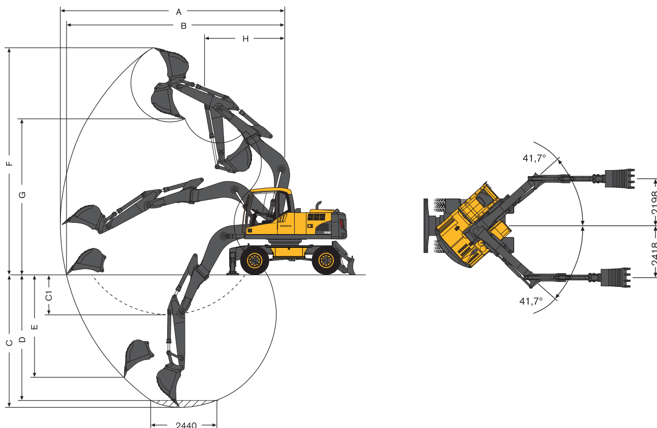
Flèche à désaxage monobloc 4,75 m et balancier 2,0 m, 2,45 m, 2,6 m, 3,1 m
